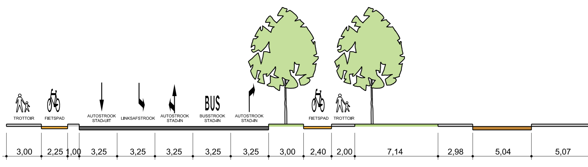
dwarsprofiel 1: Sontweg schaal 1: 200
